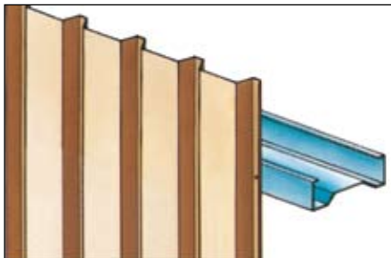
ATLAS-Clad-Wand ACW 35/0. Einschaliges Wandsystem, im Allgemeinen ohne Wärmedämmung. Paneelbefestigung an den Wandriegeln von außen durch Edelstahl-Bohrschrauben mit EPDM-Dichtung, Abdeckung der Schraubenköpfe mit Kunststoffkappen in Wandfarbe.
