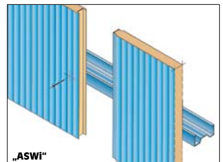
ATLAS-Sandwich-Wand ASWiP/ASWi. Verbundelemente mit wahlweise drei unterschiedlichen äußeren Oberflächenstrukturen. PU-Schaumkern für hohe Wärmedämmung und gleichzeitig homogene Verbindung zwischen Außen- und Innenschale. Befestigung an den Wandriegeln mit Edelstahl-Bohrschrauben. Stoßverbindung wie Nut- und Federsystem. Technisch einwandfreie Verbindung durch werkseitig eingebrachte Doppeldichtung.
