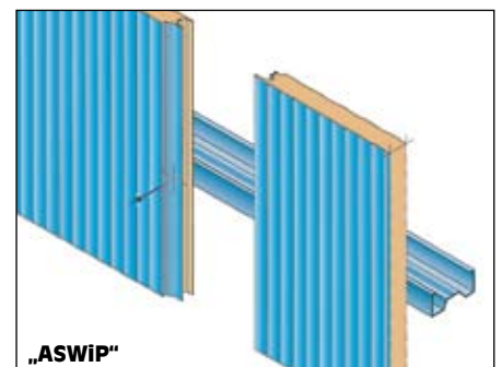
ATLAS-Clad-Wand ACW 35/75 und 100. Zweischaliges Wandsystem. Zwischen Außen- und Innenpaneel 50 mm hohes Z-Profil thermisch getrennt mit der Unterkonstruktion verschraubt. Zwischenraum für Mineralfaser-Wärmedämmung 80 bzw. 100 mm. Paneelbefestigung von außen an den Distanzprofilen durch Edelstahl-Bohrschrauben mit EPDM-Dichtung. Abdeckung der Schraubenköpfe mit Kunststoffkappen in Wandfarbe.
