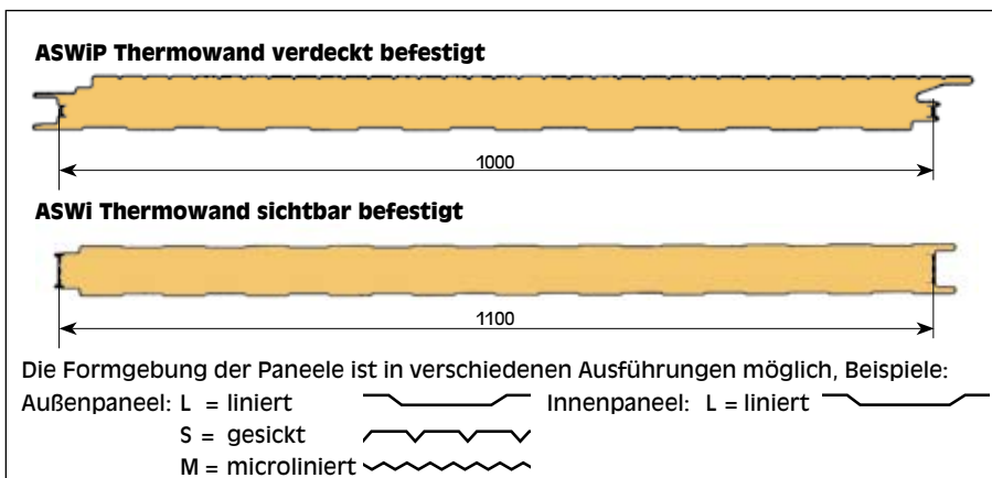
ATLAS-Sandwich-Wand ASWiP/ASWi. Verbundelemente mit wahlweise drei unterschiedlichen äußeren Oberflächenstrukturen. PU-Schaumkern für hohe Wärmedämmung und gleichzeitig homogene Verbindung zwischen Außen- und Innenschale. Befestigung an den Wandriegeln mit Edelstahl-Bohrschrauben. Stoßverbindung wie Nut- und Federsystem. Technisch einwandfreie Verbindung durch werkseitig eingebrachte Doppeldichtung.
