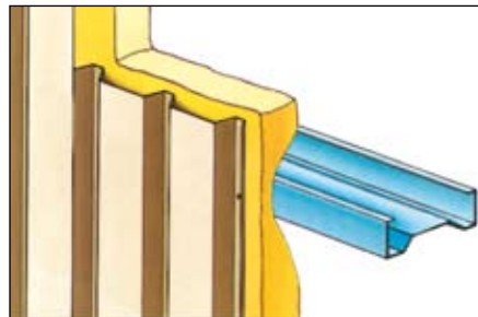
ATLAS-Clad-Wand ACW 35/0i. Einschaliges Wandsystem mit folienkaschierter Mineralfaser-Wärmedämmung bis 80 mm zwischen Paneel und Wandriegel. Paneelbefestigung an den Wandriegeln von außen durch Edelstahl-Bohrschrauben mit EPDM-Dichtung. Abdeckung der Schraubenköpfe mit Kunststoffkappen in Wandfarbe.
