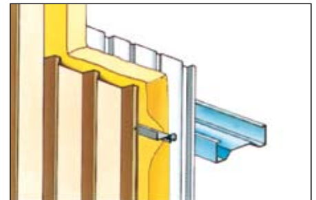
ATLAS-Clad-Wand ACW 35/75 und 100. Zweischaliges Wandsystem. Zwischen Außen- und Innenpaneel 50 mm hohes Z-Profil thermisch getrennt mit der Unterkonstruktion verschraubt. Zwischenraum für Mineralfaser-Wärmedämmung 80 bzw. 100 mm. Paneelbefestigung von außen an den Distanzprofilen durch Edelstahl-Bohrschrauben mit EPDM-Dichtung. Abdeckung der Schraubenköpfe mit Kunststoffkappen in Wandfarbe.
