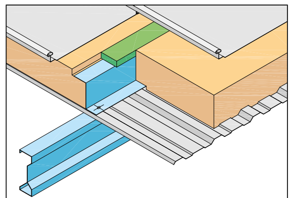
ATLAS-Eurorib-Dach AER 60/80 bis 160. Zweischaliges Dachsystem, Ständersystem zwischen Außen- und Innenpaneel, mit der Unterkonstruktion verschraubt. Zwischenraum für die Mineralfaser-Wärmedämmung 80, 100, 120, 140 und 160 mm. 30 mm dicker Thermoblock zur Vermeidung von Wärmebrücken zwischen Pfette und Dachpaneel. Verdeckt liegende Befestigung. Kraftschlüssige Verbindung und Dichtung der Stehfalzränder durch maschinelle Verbördelung.
