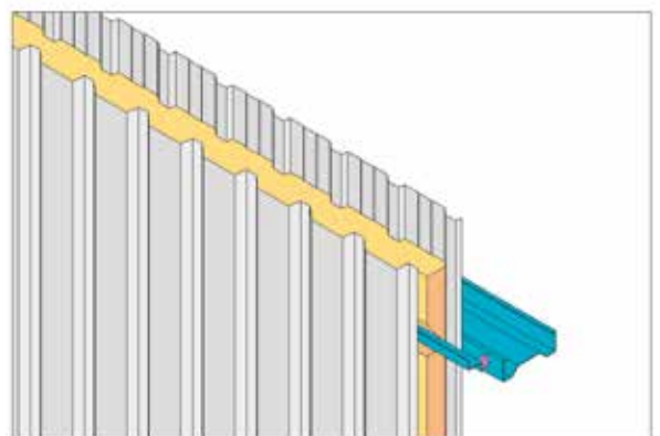
ATLAS-Clad-Wand ACW 35/75 und 100. Zweischaliges Wandsystem. Zwischen Außen- und Innenpaneel 50 mm hohes Z-Profil thermisch getrennt mit der Unterkonstruktion verschraubt. Zwischenraum für Mineralfaser-Wärmedämmung 80 bzw. 100 mm. Paneelbefestigung von außen an den Distanzprofilen durch Edelstahl-Bohrschrauben mit EPDM-Dichtung. Abdeckung der Schraubenköpfe mit Kunststoffkappen in Wandfarbe.
