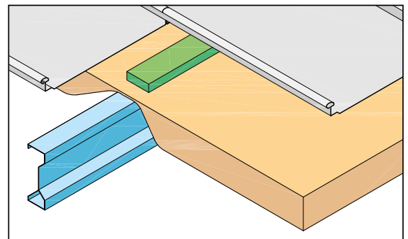
ATLAS-Eurorib-Dach AER 60/30. Einschaliges Dachsystem, mit Mineralfaser-Wärmedämmung, Dicke 100 bis 120 mm. Zur Vermeidung von Wärmebrücken zwischen Pfette und Dachpaneel 30 mm dicker Thermoblock. Verdeckt liegende Befestigung. Kraftschlüssige Verbindung und Dichtung der Stehfalzränder durch maschinelle Verbördelung.
