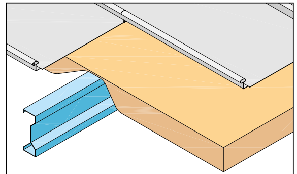
ATLAS-Eurorib-Dach AER 60/0i. Einschaliges Stehfalz-Dachsystem ohne oder mit Mineralfaser-Wärmedämmung ausführbar. Dicke der Mineralfasermatte bis max. 80 mm, vorwiegend als Tropfschutz. Verdeckt liegende Befestigung. Kraftschlüssige Verbindung und Dichtung der Stehfalzränder durch maschinelle Verbördelung.
