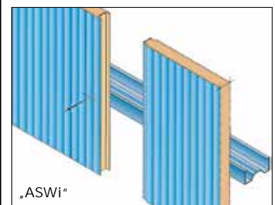
ASWi-Thermowand sichtbar befestigt
