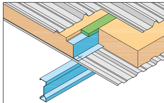
ATLAS-Clad-Dach ACR 40/80 bis 160.
